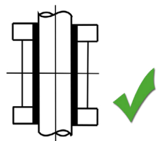
Buchsen mit Doppelkonus
