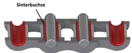
Kette LUB FREE VERTE
