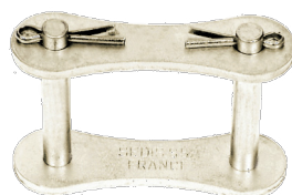
N°208 : Maillon de jonction goupillé
