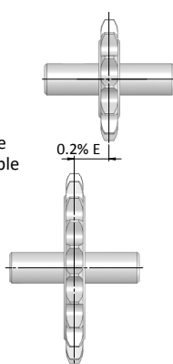
tolérance d'alignement
