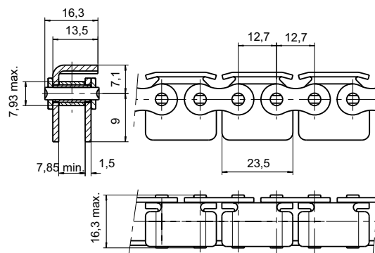
Chaîne 40 "Type KC" (5415-08) Résistance à la traction mini = 16.5 kN
