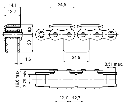
Chaîne 7N "Type KC" (5272-70) Résistance à la traction mini = 18.2 kN
