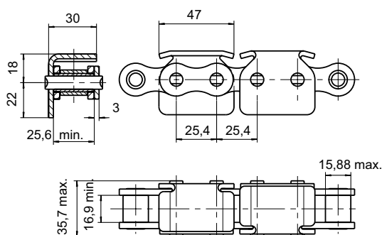
Chaîne 15T "Type KC" (5288-03) Résistance à la traction mini = 66 kN
