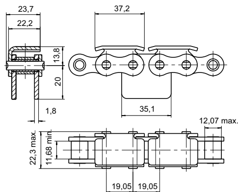
Chaîne 13N "Type KC" (5268-27) Résistance à la traction mini = 30.5 kN
