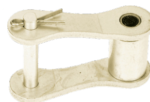
N°216 : Maillon coudé simple goupillé
