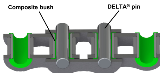
DELTA® VERTE chain
