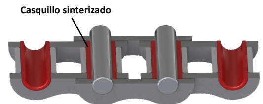
Cadena LUB FREE VERTE
