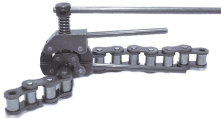
Extractor de eje de cadenas réf 9160
