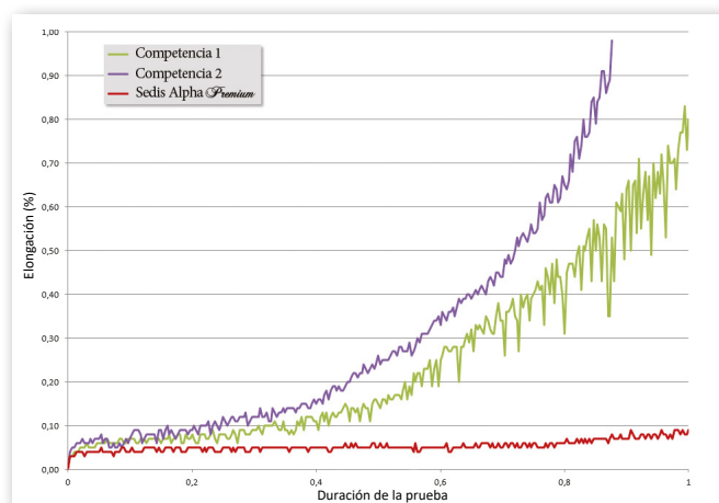
Desgaste de una cadena ASA 50-1 Alpha Premium SEDIS comparada a 2 cadenas competidoras
