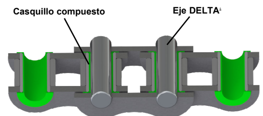
Cadena DELTA® VERTE
